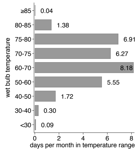
(D) Wet bulb temperature density
